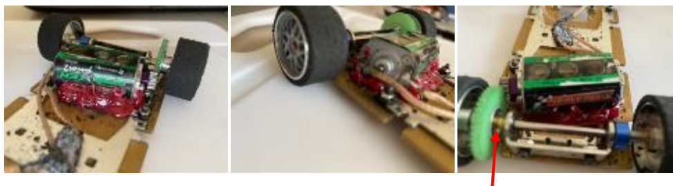
Eje trasero macizo (por seguridad opino que en esta categoría es mejor no emplear los ejes huecos atrás) de Sigma de 65 mm (no es necesaria una mayor anchura, ya que las llantas traseras tienen 13 mm de anchura cada una).
